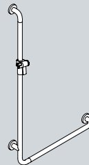
Vinkelhåndtak med dusjholder 805.33.210 Horisontal lengde 400, H 1100, D 90, ø 33
