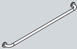
Støtthåndtak 802.36.140 Senteravstand 900, D 90, ø 33
