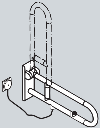
HC-støtte med spyleknapp (elektr.) 801.50.750 B 78, H 259, L 700
