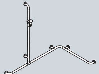
Dusjstøtthåndtak med skyvbar dusjholder 802.35.300 B 1185 x 762, H 1100, D 90, ø 33
