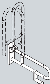
HC-støtte 801.50.1... Veggplate B 78, H 259 ...00 L 600 ...10 L 700 ...20 L 850 Oppgraderingssett toalett- papirholder 801.50.010
