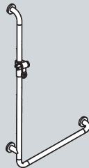
Vinkelhåndtak med dusjholder 801.33.210 Senteravstand 600, H 1100, D 90
