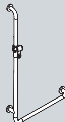
Vinkelhåndtak med dusjholder 802.33.210 Horisont. lengde 600, H 1100, D 90, ø 33
