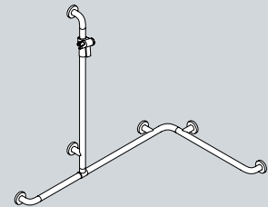
Dusjstøttehåndtak med dusjholder 805.35.300 B 1185 x 762, H 1100, D 90, ø 33
