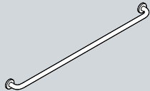
Støttehåndtak 805.36.1... Stang ø 33 Rosetter ø 70 Senteravstand: ...00 Senteravstand 300 ...10 Senteravstand 400 ...20 Senteravstand 500 ...30 Senteravstand 600 ...40 Senteravstand 900 ...50 Senteravstand 1100
