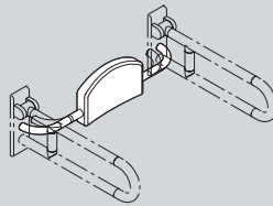
Ryggstøtte 801.51.900 B 670-730, H 220, D 150
