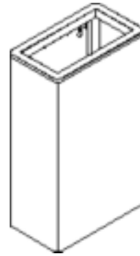
Avfallskurv* Paper towel basket 805.05.100 300 | 510 | 170
