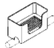
Oppbevaringsboks Storage box 802.03.200 200 | 110 | 107
